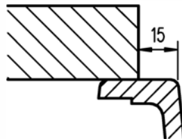
Detail 1:2
